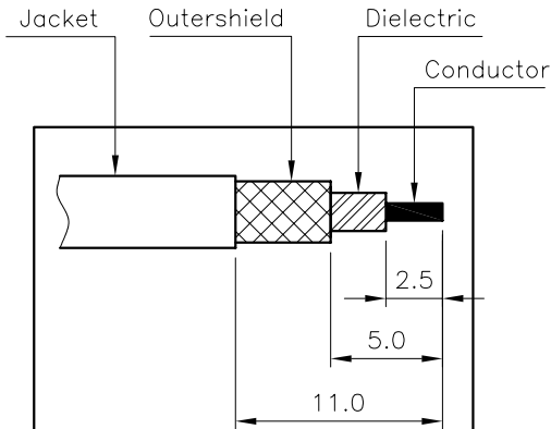
2번 커넥터 탈피도
