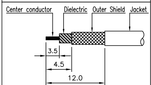
3번 CONNECTOR 탈피도
