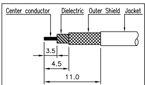
2번 CONNECTOR 탈피도
