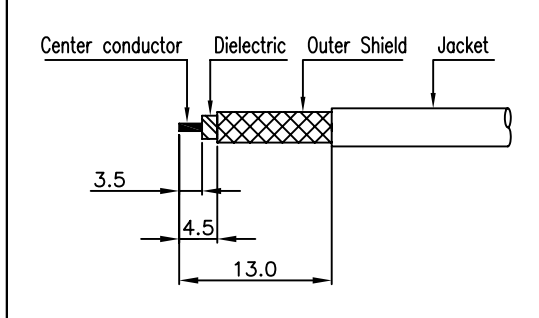
3번 커넥터 케이블 탈피도
