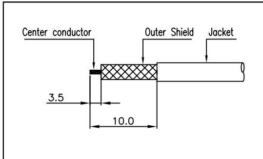
2번 커넥터 케이블 탈피도
