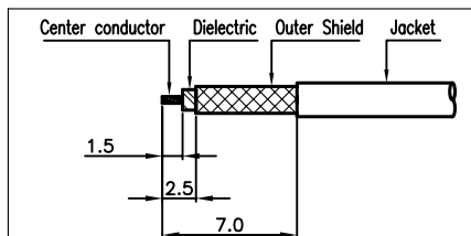
2번 커넥터 케이블 탈피도
