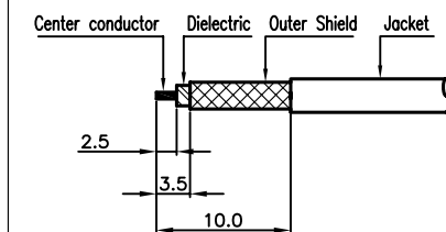
3번 커넥터 케이블 탈피도
