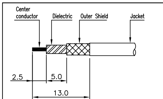
2번 커넥터 케이블 탈피도
