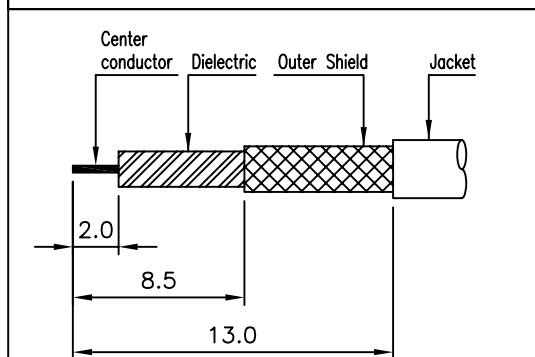
3번 커넥터 케이블 탈피도
