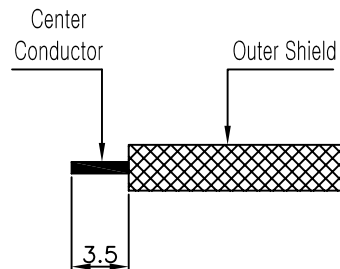
③ CABLE 탈피도
