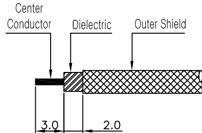
② CABLE 탈피도
