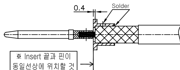
N Type 케이블 심선+핀 조립
