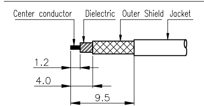
②번 Connector 탈피도
