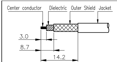
③번 Connector 탈피도
