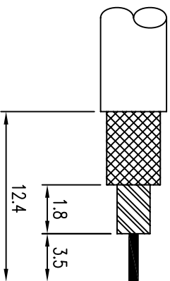
CABLE ASS'Y 탈피도
