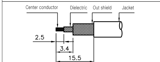
3번 CONNECTOR 탈피도
