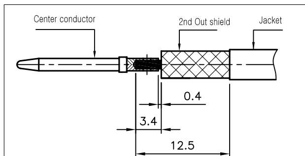
2번 CONNECTOR 탈피도
