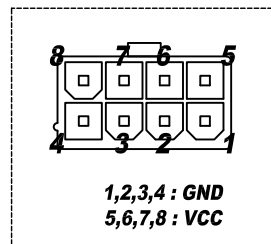
한림전자 LAD1140-8 PIN MAP
