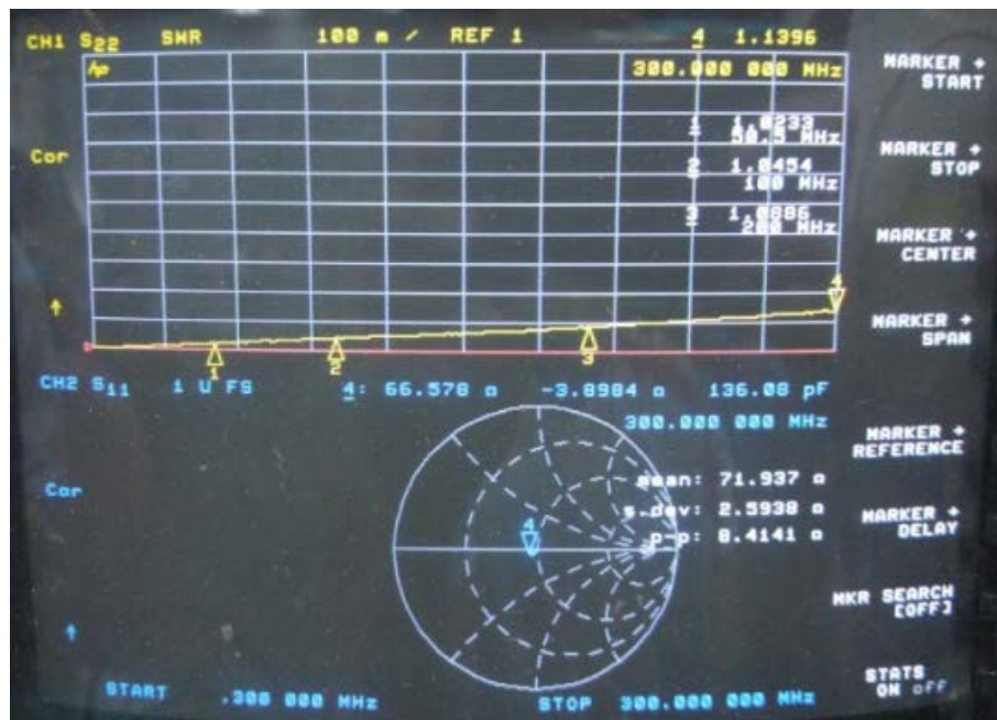
그림2) TR1 : OUT Port VSWR, TR2: Impedance
