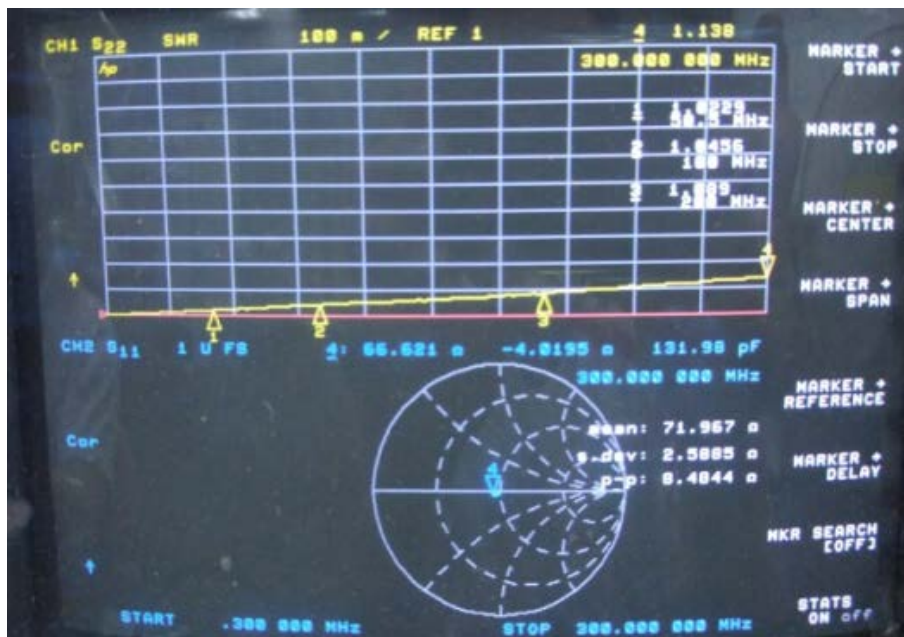
그림2) TR1 : OUT Port VSWR, TR2: Impedance
