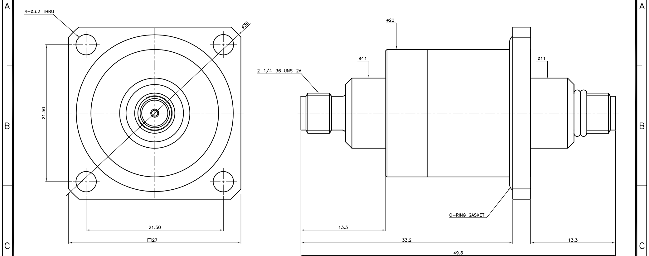
LABEL 부착 외관도
